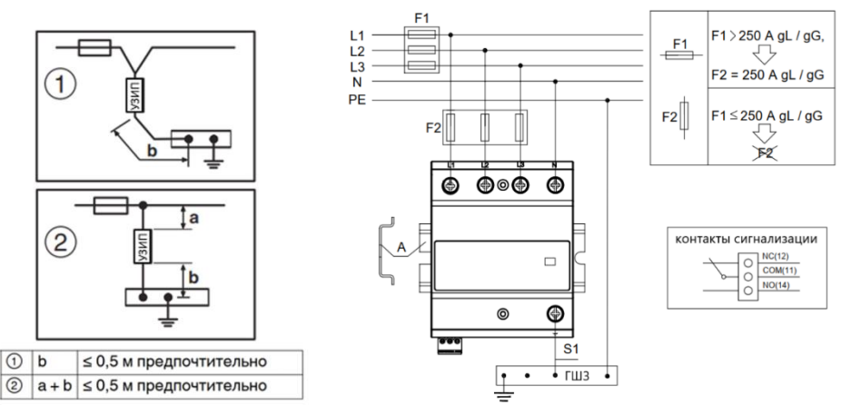
Рис.1. Варианты подключения
