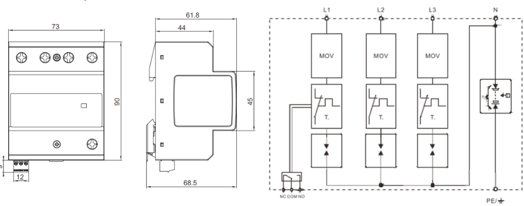
Рис.3. Габаритный чертеж
