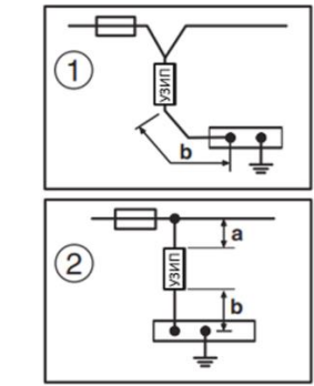
Рис.1. Варианты подключения
