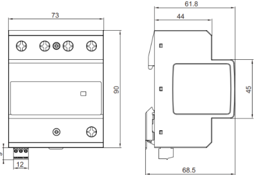
Рис.3. Габаритный чертеж
