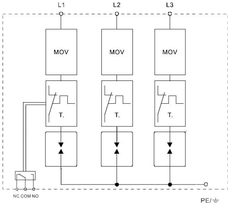
Рис.4. Схема Электрическая
