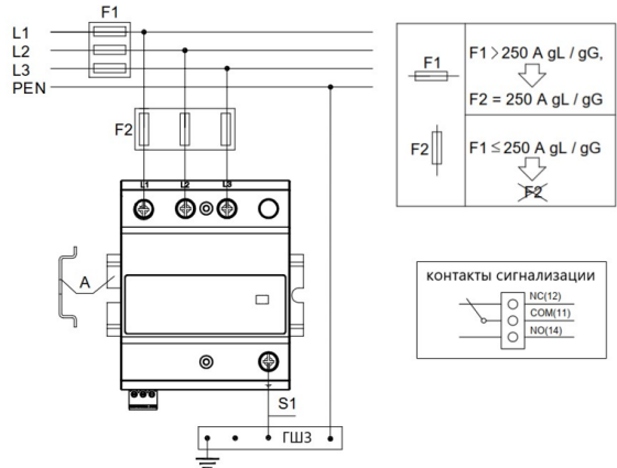
Рис.2. Схема подключения
