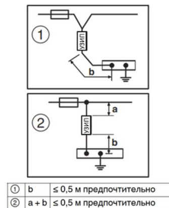
Рис.1. Варианты подключения
