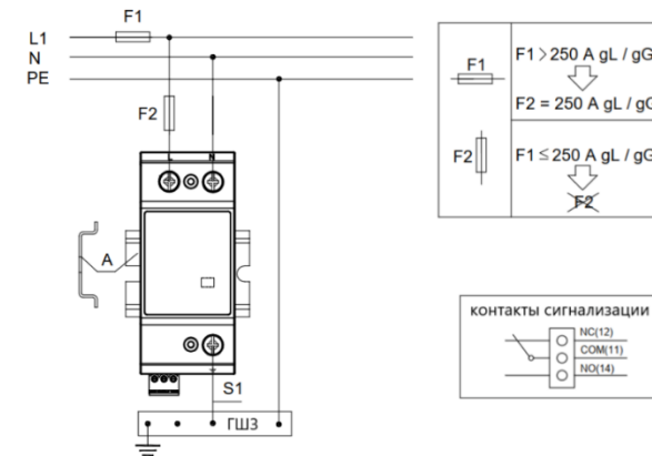
Рис.2. Схема подключения
