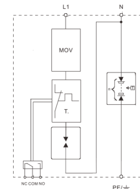
Рис.4. Схема Электрическая
