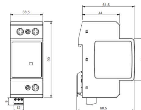
Рис.3. Габаритный чертеж
