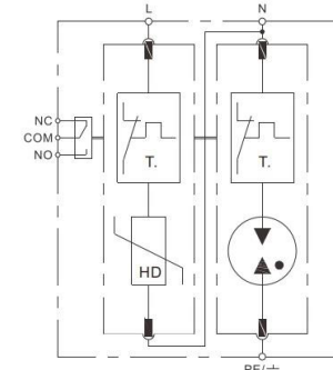
Рис.4. Схема Электрическая
