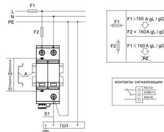
Рис.2. Схема подключения
