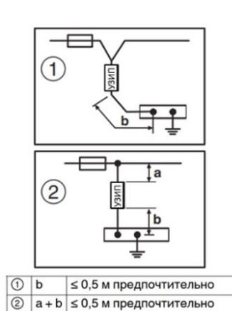
Рис.1. Варианты подключения
