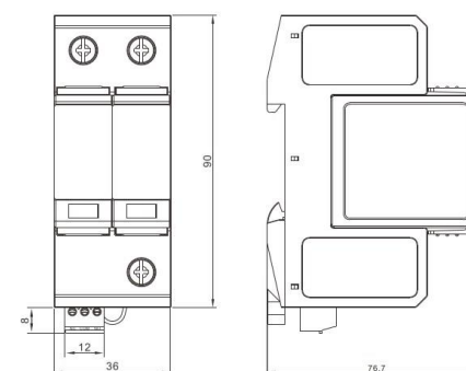
Рис.3. Габаритный чертеж
