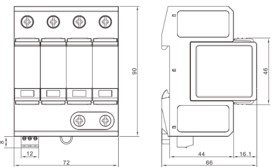
Рис.3. Габаритный чертеж
