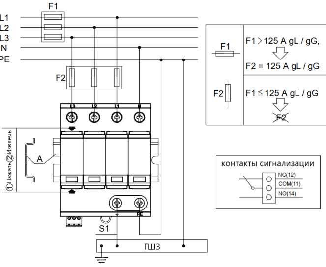
Рис.2. Схема подключения
