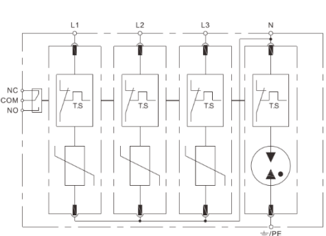
Рис.4. Схема Электрическая
