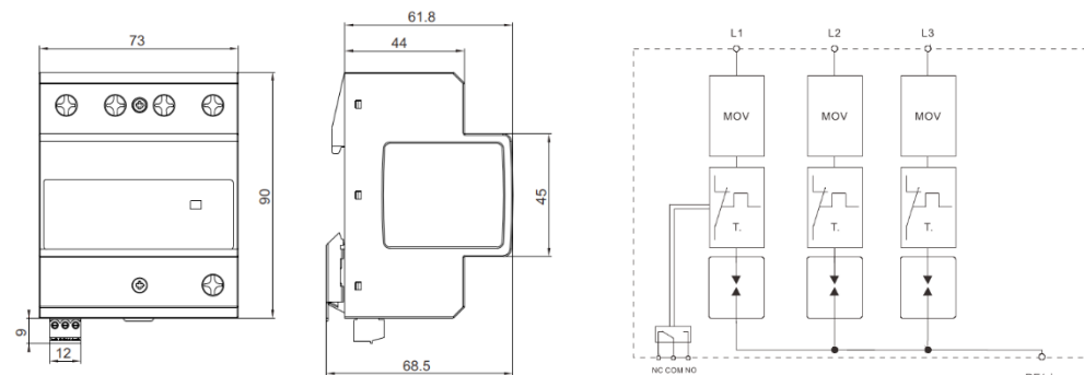
Рис.3. Габаритный чертеж
