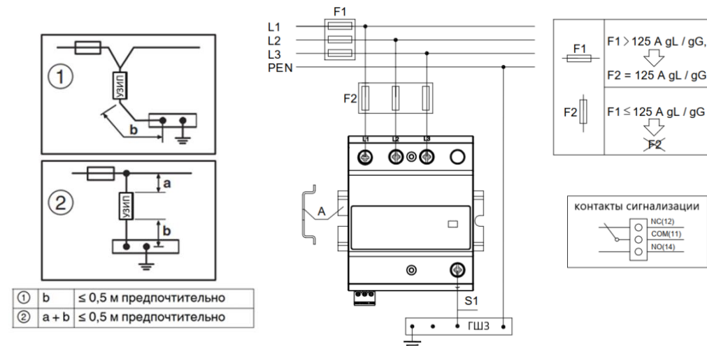
Рис.1. Варианты подключения
