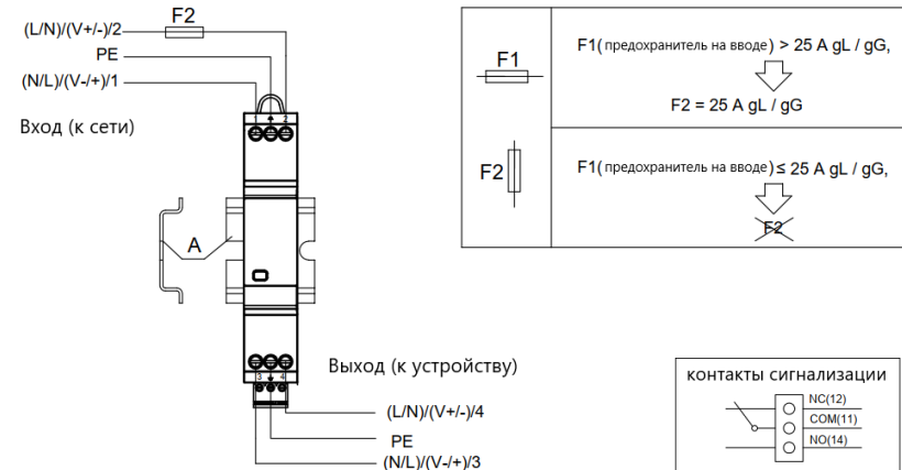
Рис.1. Схема подключения
