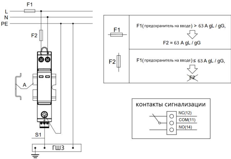
Рис.1. Схема подключения
