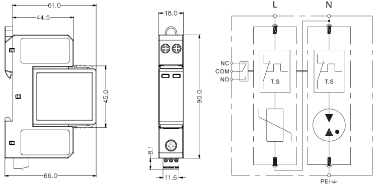
Рис.2. Габаритный чертеж
